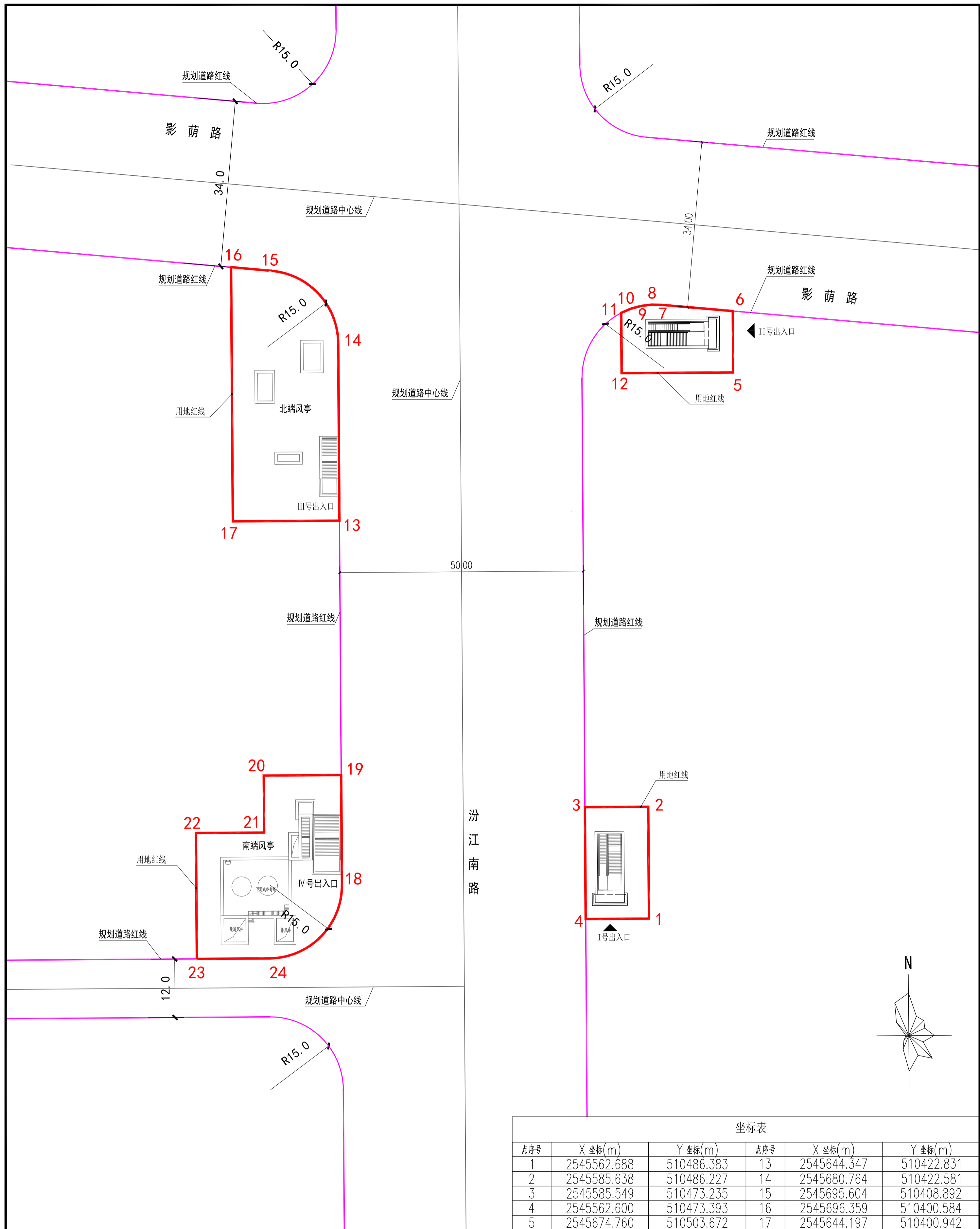
季华园站建设用地示意图 1: 500
